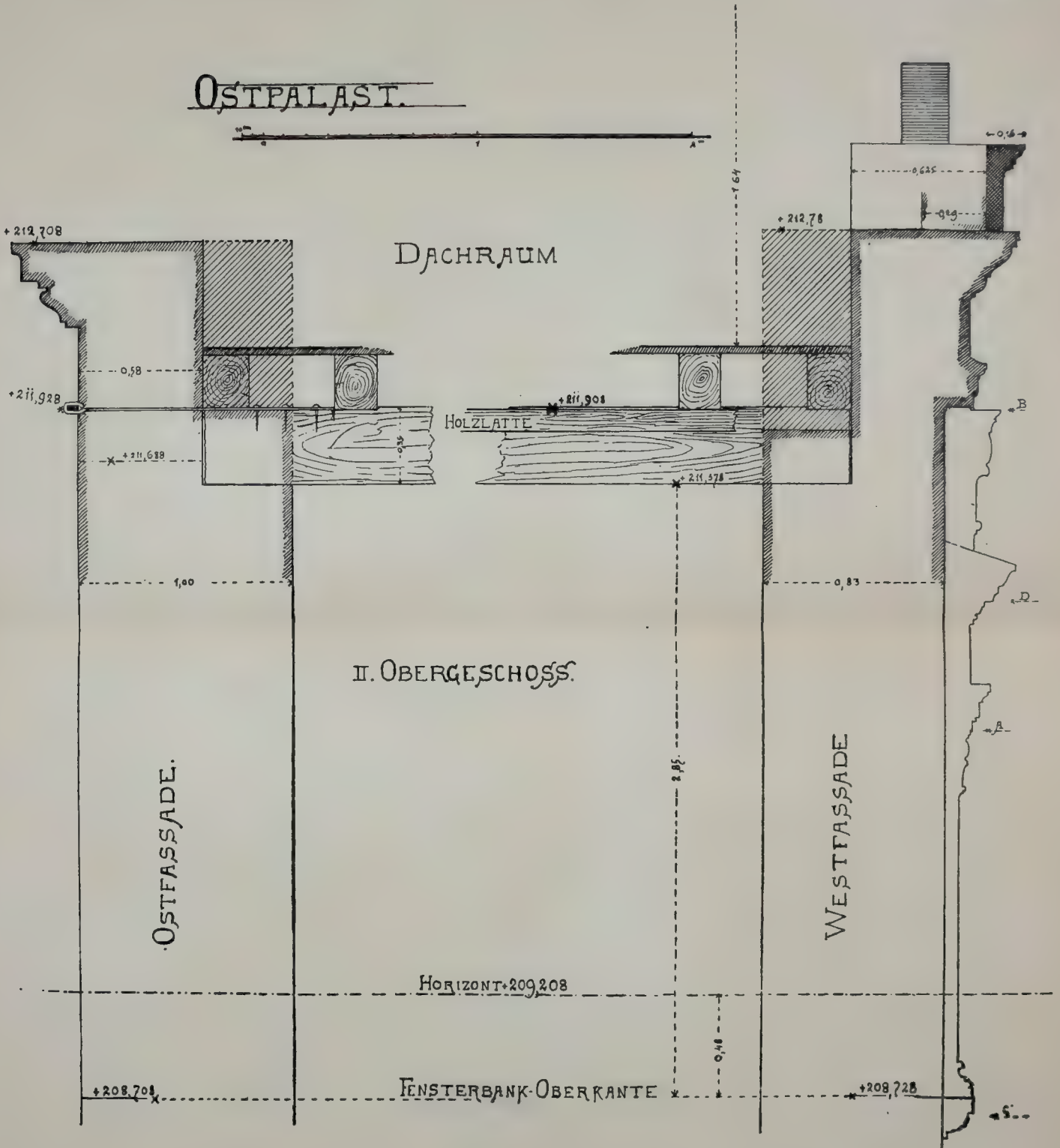
ABB. 6. QUERSCHNITT DURCH DEN OSTPALAST DES HEIDELBERGER SCHLOSSES.
